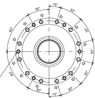
See C C矢视图 (12-M12タップ(☆印)角度詳細)
