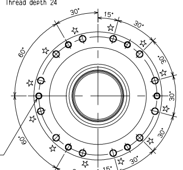
C矢視図 (12-M12タップ (☆印)角度詳細)
